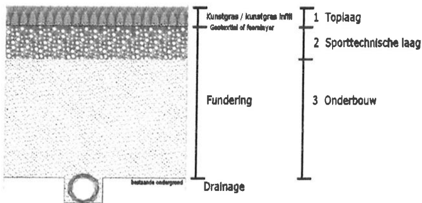
Figuur 2.1 Opbouw van een kunstgrasveld
