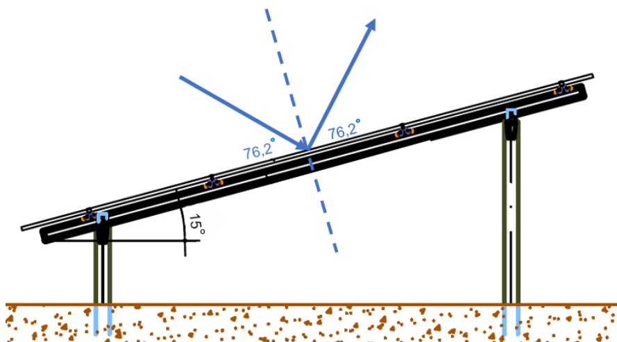
Figuur 26: Hoeken van reflectie
