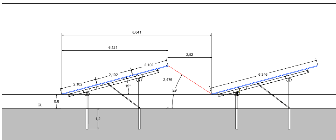
Figuur 8: Doorsnede van de opstellingen
