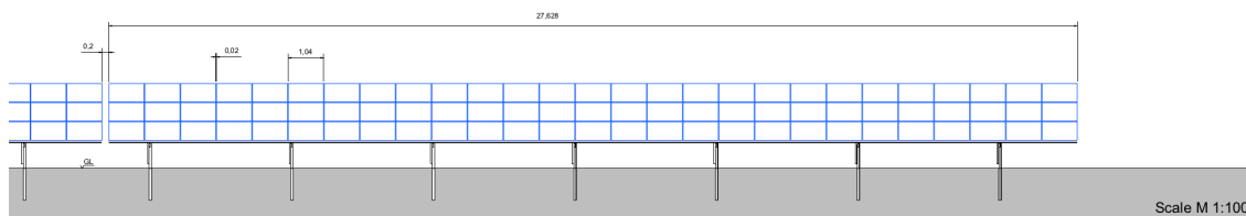
Figuur 9: Vooraanzicht opstelling van de panelen
