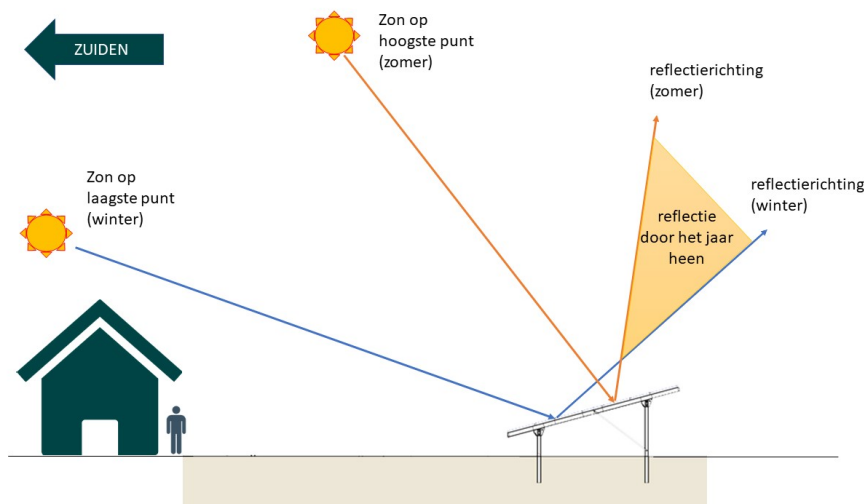
Figuur 25: Lichtweerkaatsing op zonnepanelen
