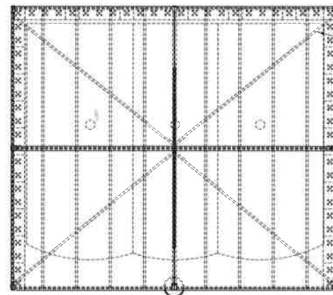
Windverband
