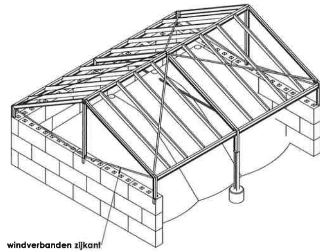
windverbanden zijkant
