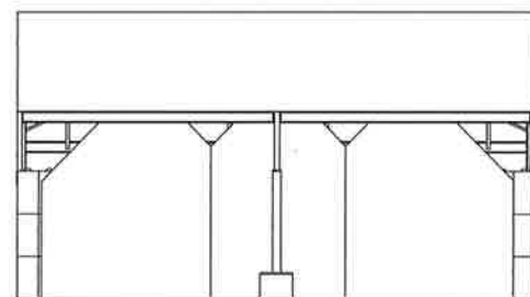
Afgedekte overkapping constructie op wanden van Lego stapel betonblokken. Verankering aan 3 zijden aan betonblokken constructie in overleg met constructeur
