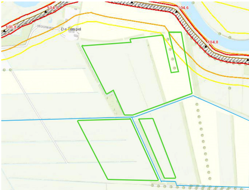
Figuur 24: Waterkering (rood) met primaire (oranje) en secundaire (geel) beschermingszone, en primaire watergangen sw20.4 en SW20.66 (blauw), met in groen de grenzen van de te bebouwen gebieden
