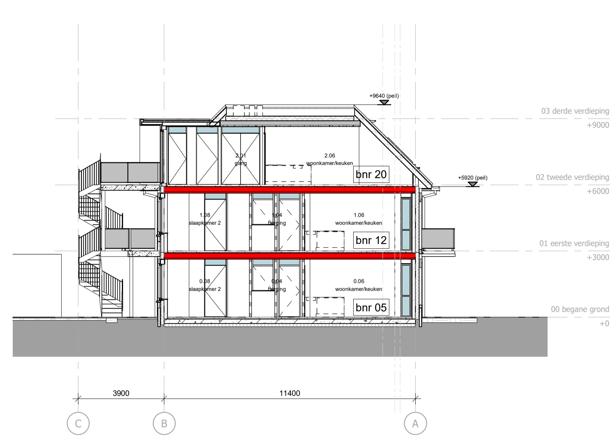
doorsnede B-B
