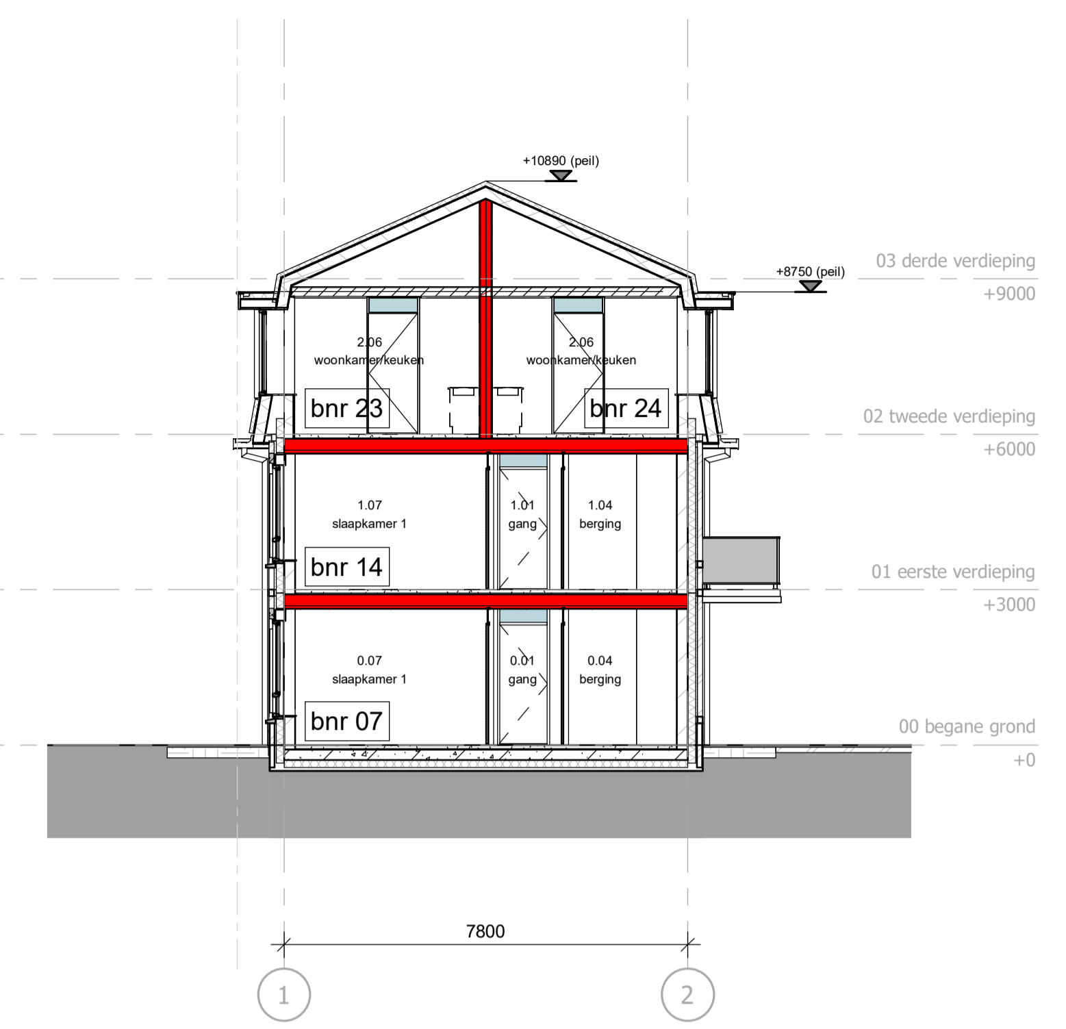
doorsnede C-C
