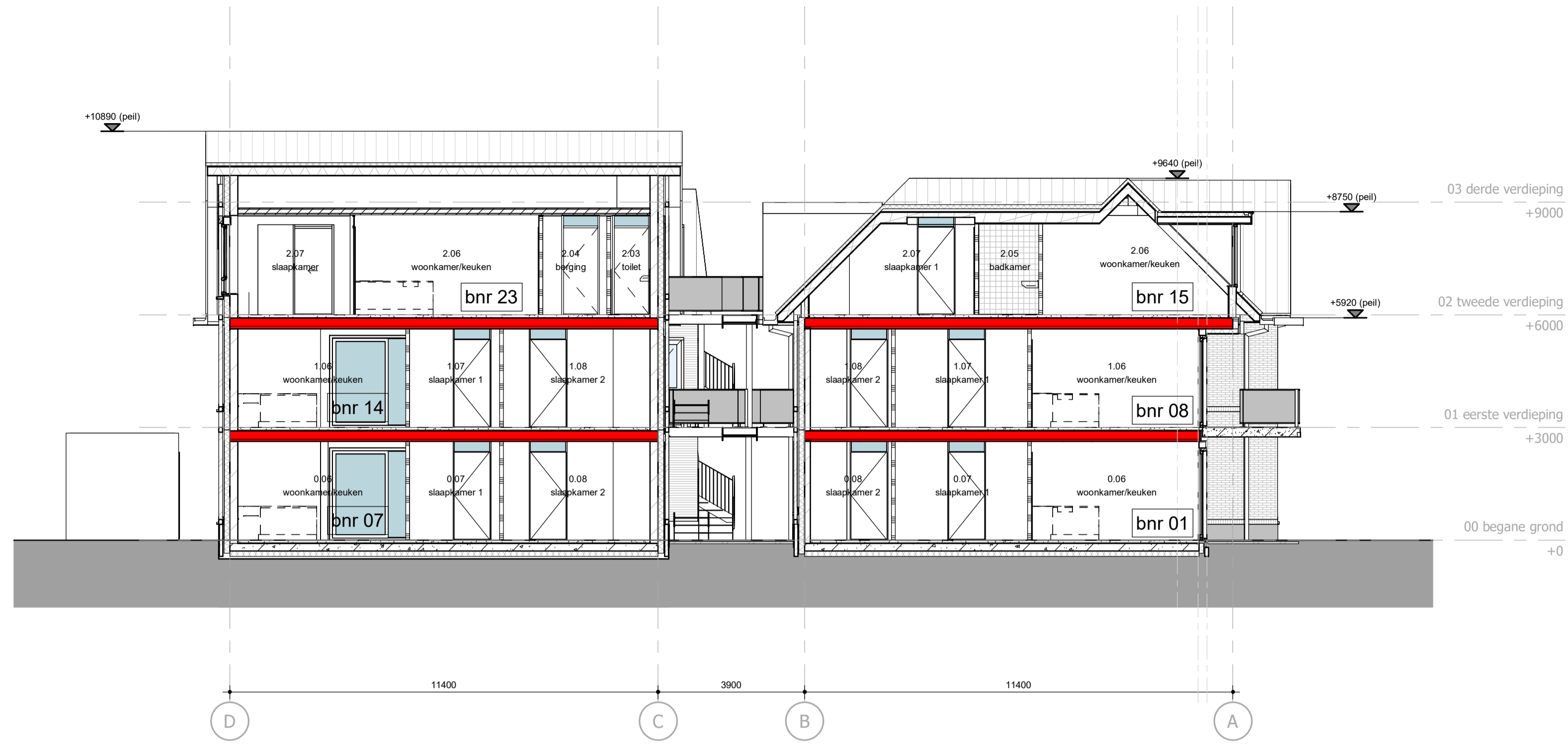
doorsnede A-A
