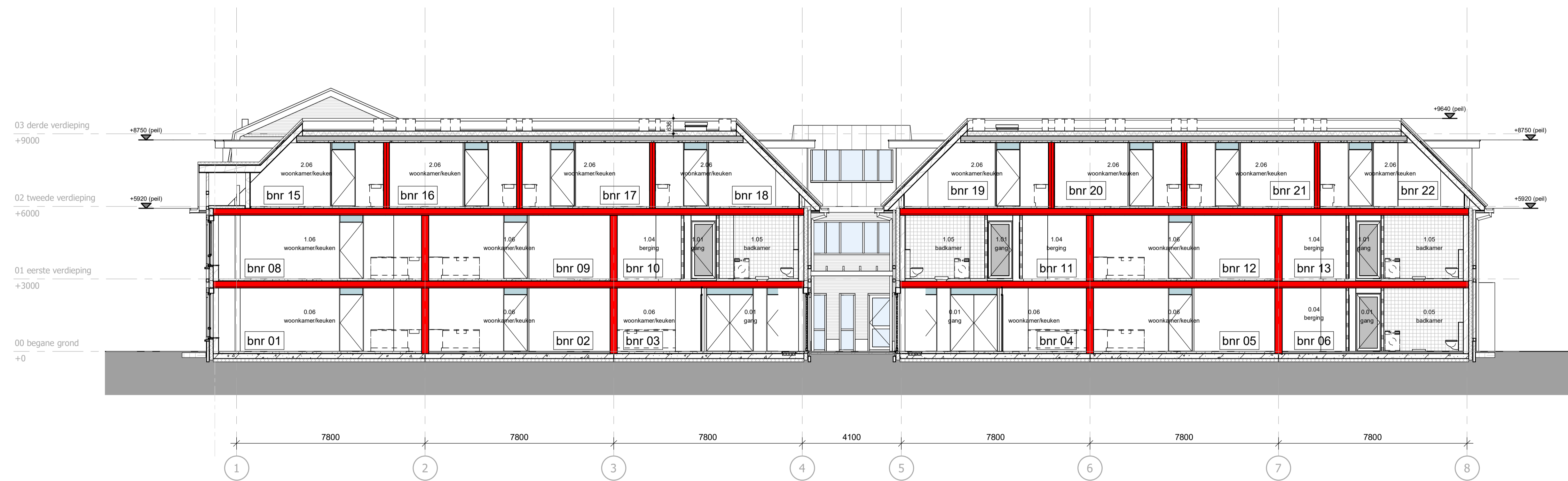
doorsnede D-D
