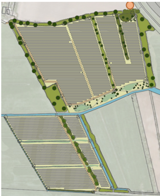
Uitsnede landschapsschets zonnepark
