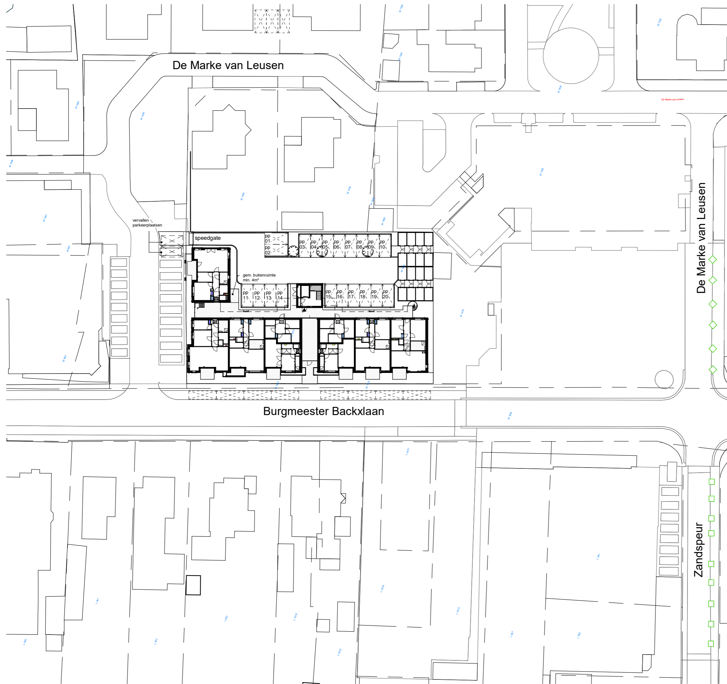
situatie - nieuw
