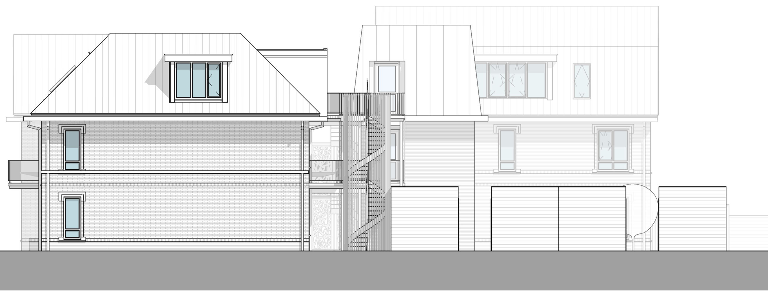
rechter gevel
